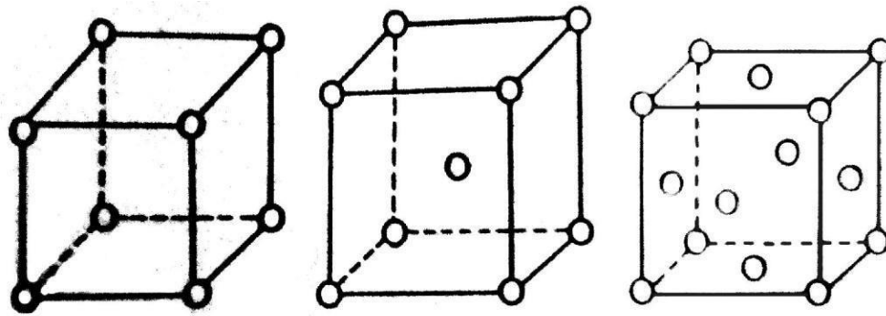
Simple cubic
